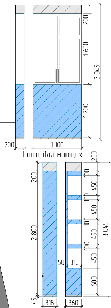
Зашивка инсталляции h=1200мм
