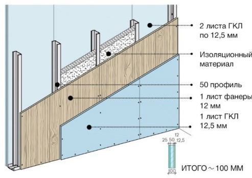
Узел усиленной перегородки
